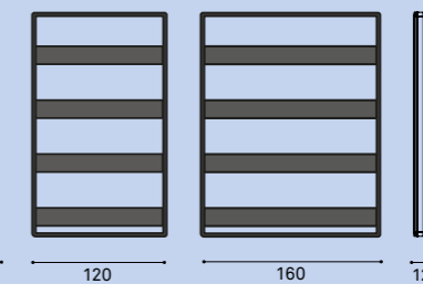
planter trays h 15 x d 12 cm (4 pieces) / Pflanzentröge h 15 x t 12 cm (4 Stück)
